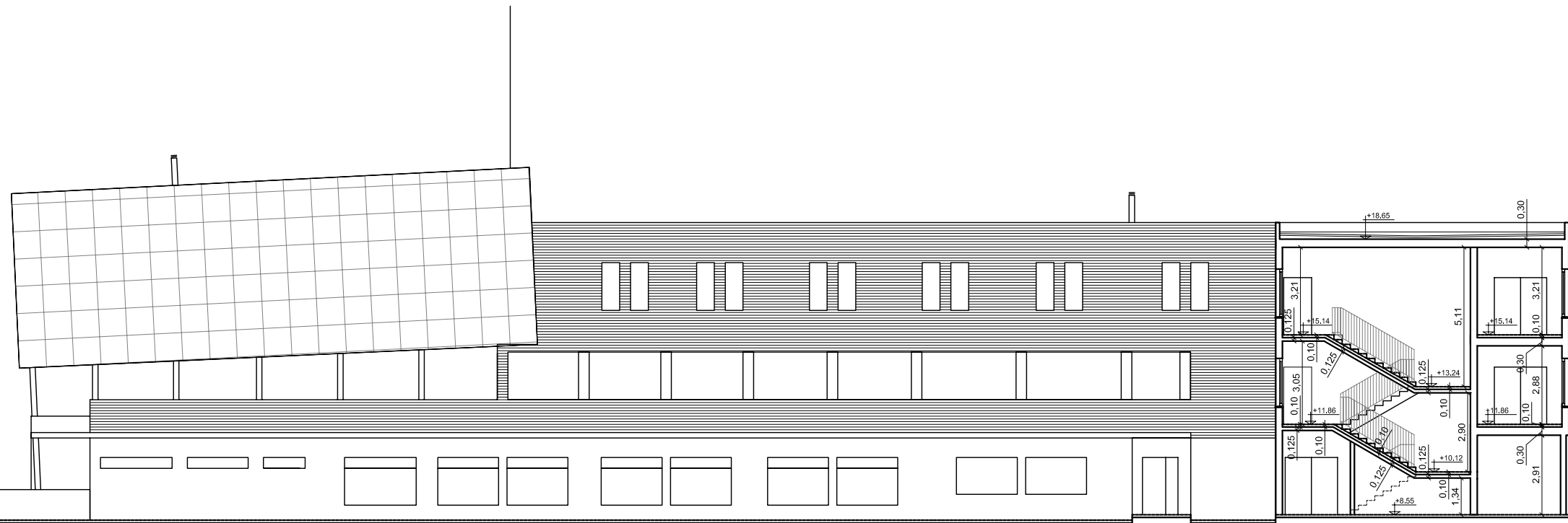
SECCIÓN 2-2
