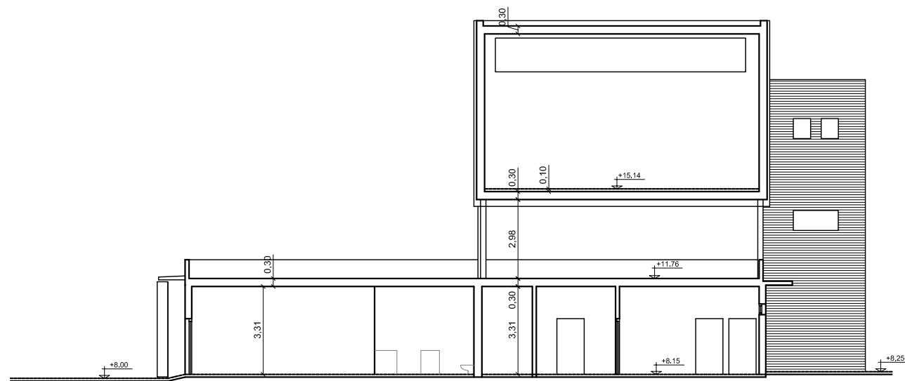
SECCIÓN 3-3
